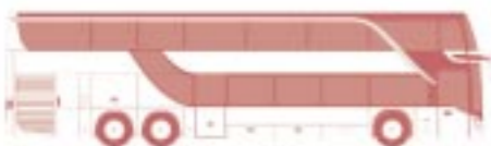
S 431 DT, Länge 13 890 mm
